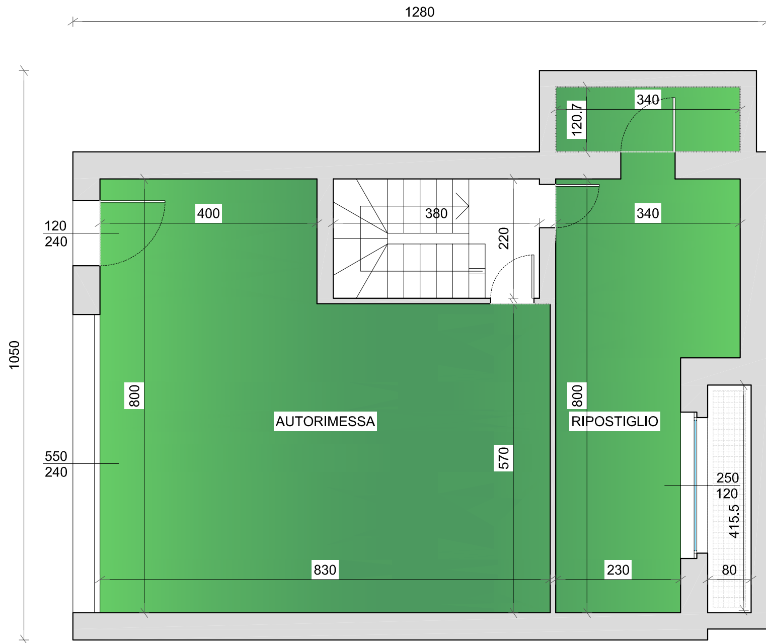
VILLA DALIA PIANTA PIANO INTERRATO Autorimessa 56.50 mq Ripostiglio 22.00 mq
